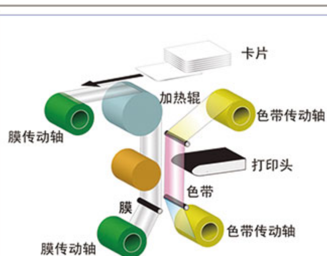
Prima 4 证卡打印机工作原理
