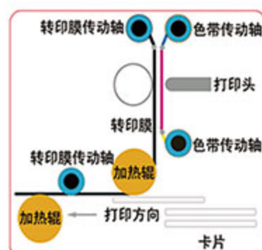
卡片弯曲矫正模块工作原理
