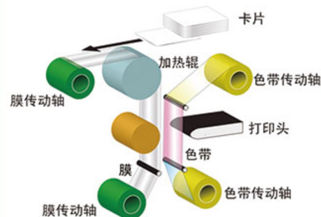
CX7000证卡打印机工作原理
