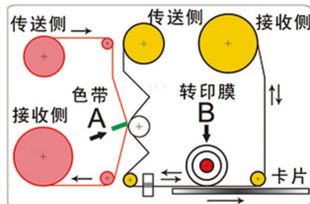
P55打印原理示意图
